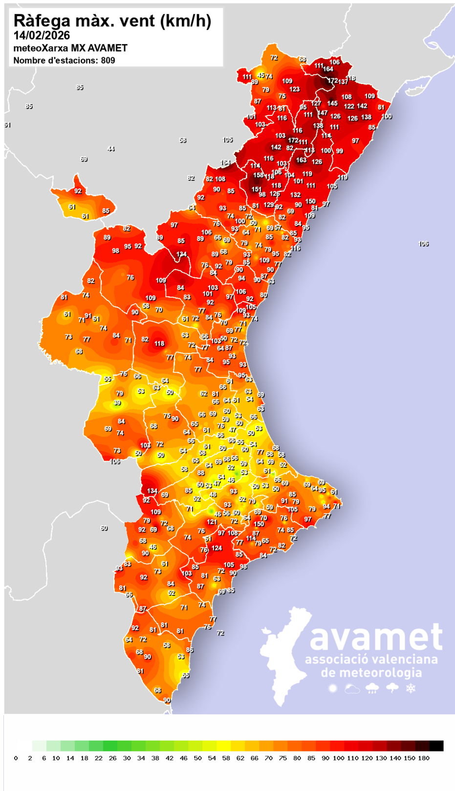
Figura 4. Mapa de racha máxima de viento el 14/02/2026. Fuente: AVAMET.
